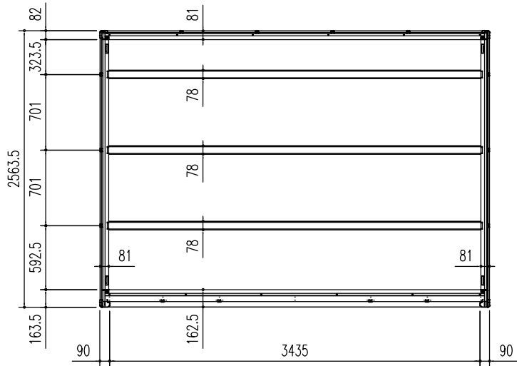
床 伏 図 (S = 1/50)
