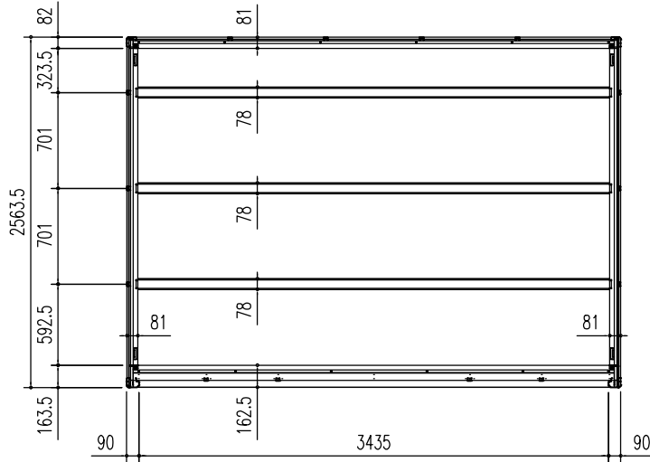
床 伏 図 (S = 1/50)
