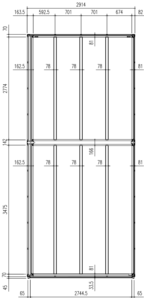
床伏図 (S=1/50)
