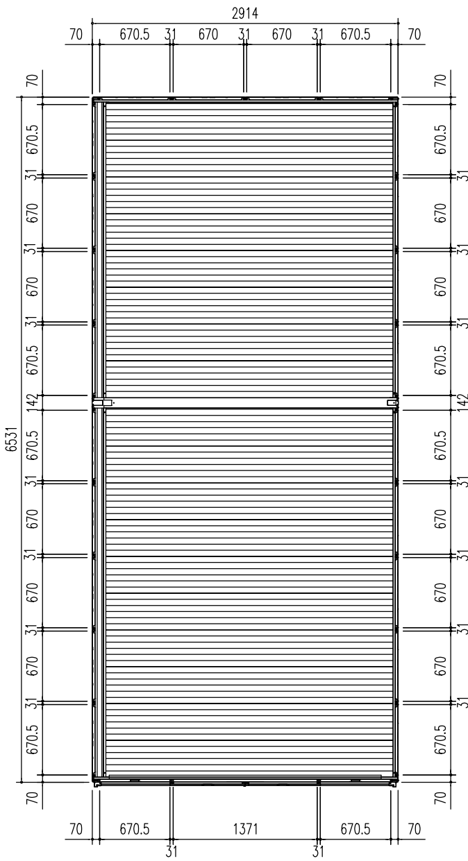
平面図 (S=1/50)
