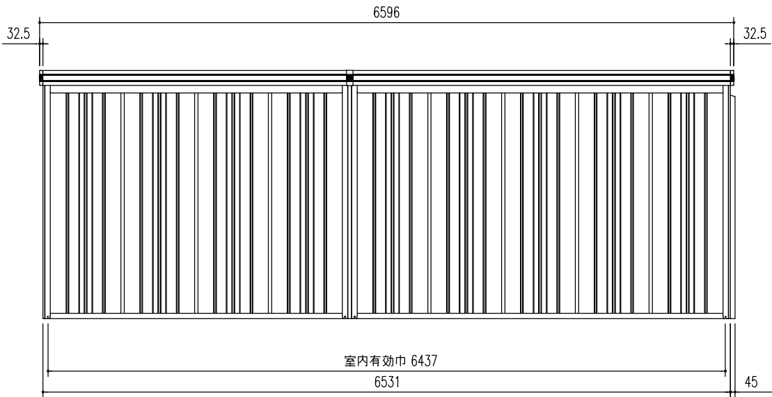
側面立面図 (S=1/50)
