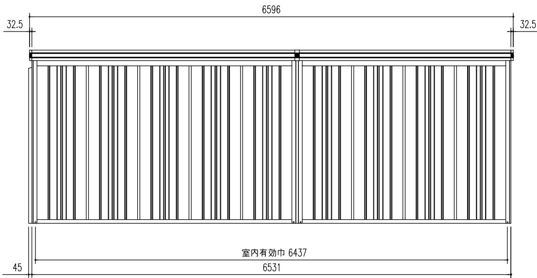
側面立面図 (S=1/50)
