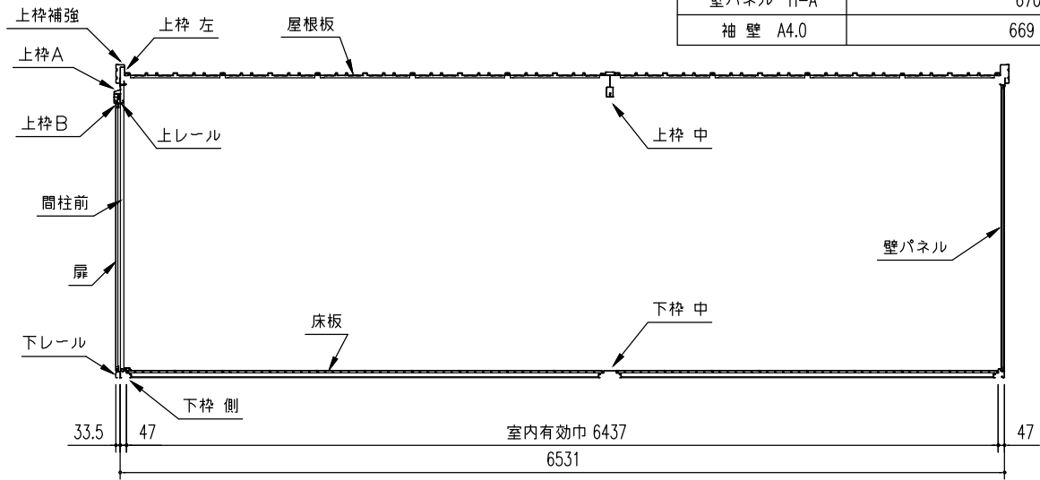
側面断面図 (S=1/50)
