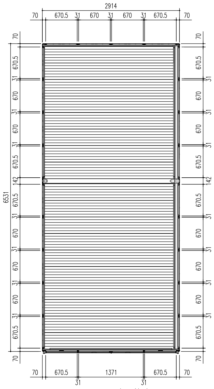
平面図 (S=1/50)
