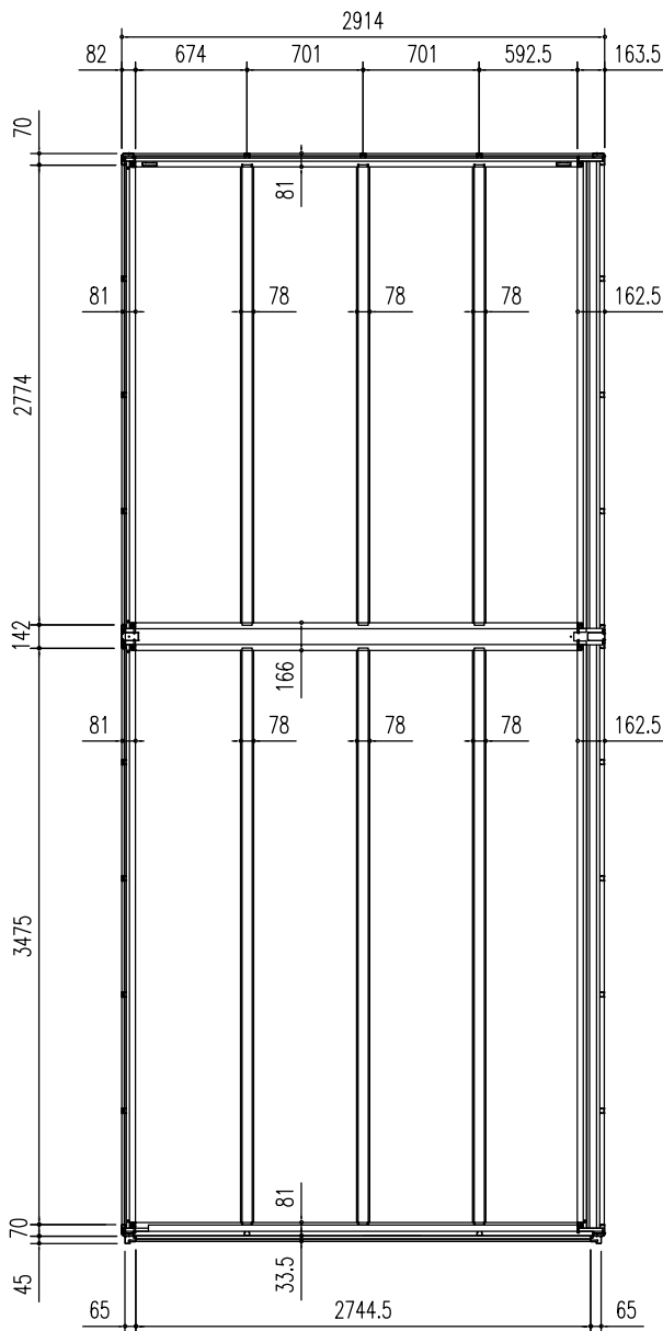
床伏図 (S=1/50)
