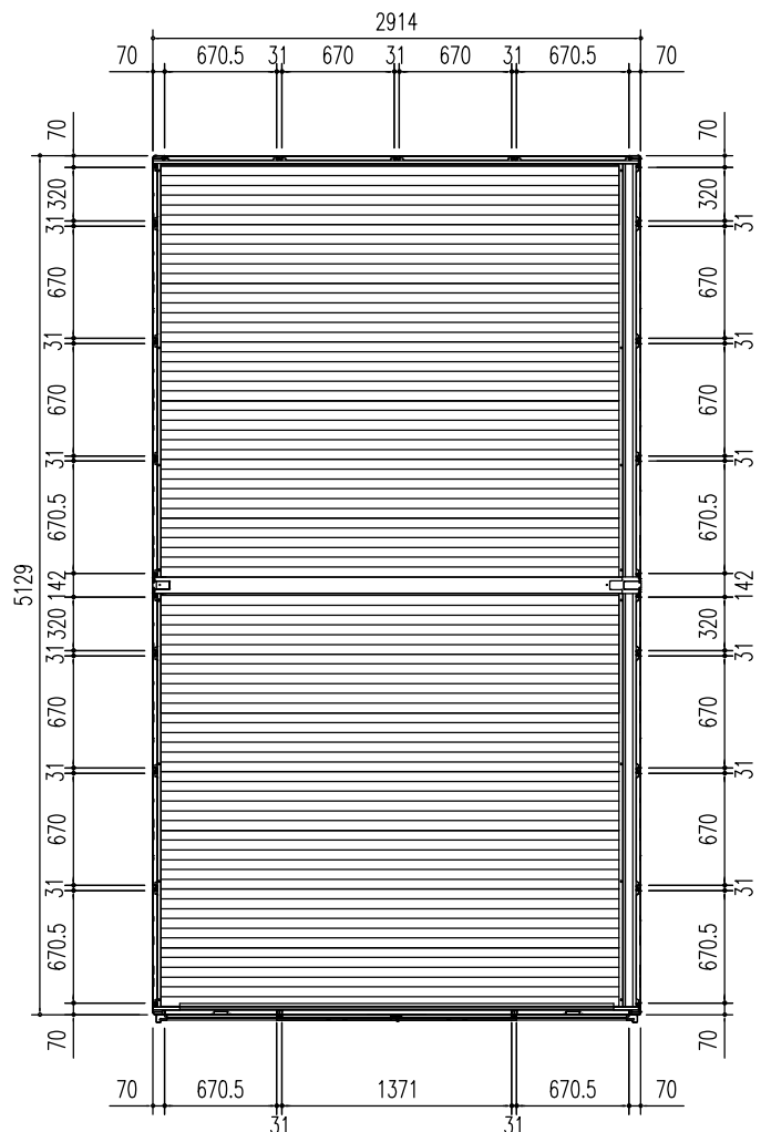
平面図 (S=1/50)
