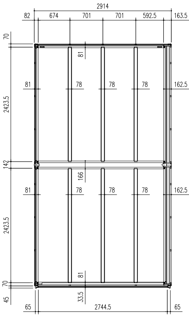
床伏図 (S=1/50)
