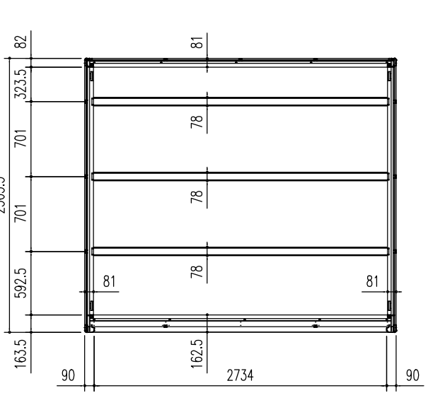
床伏図 (s = 1/50)
