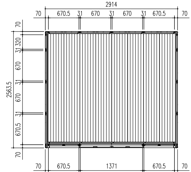
平面図 (s = 1/50)
