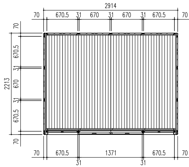
平面図 (S = 1/50)
