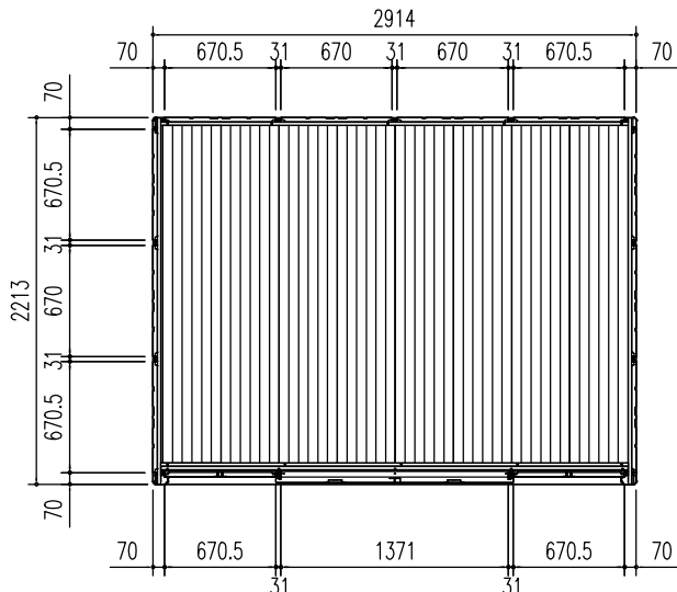
平面図 (S = 1/50)
