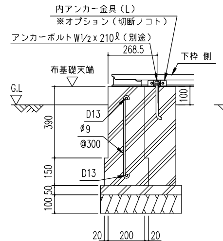
D ~ D' 断 面
