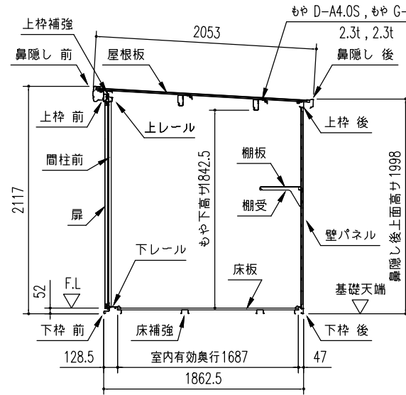
積雪型矩計図 (S = 1/50)
