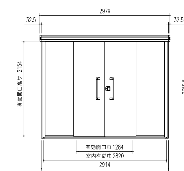
正面立面図 (S = 1/50)
