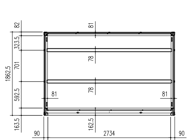
床 伏 図 (S = 1/50)
