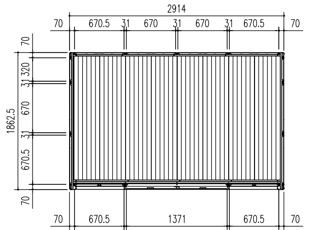
平面図 (S = 1/50)
