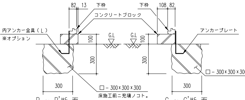
B ~ B'断面 (内アンカー用)
