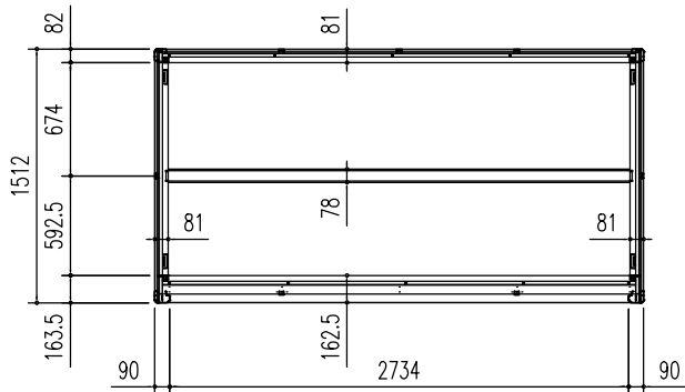
床伏図 (S=1/50)
