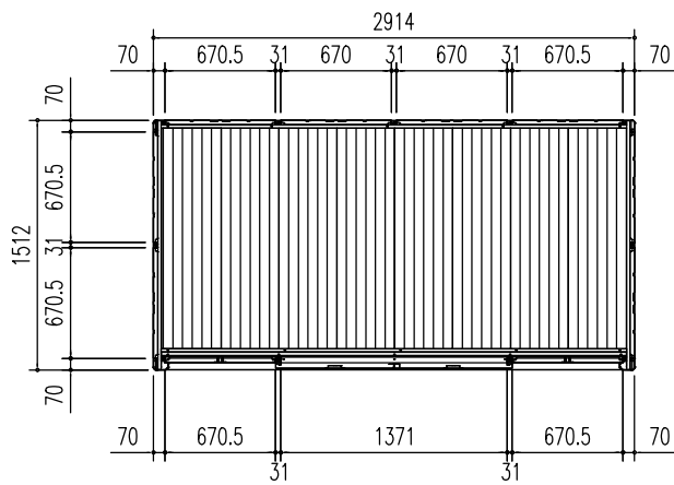
平面図 (S=1/50)
