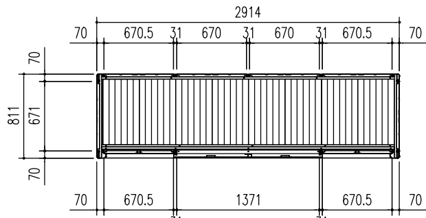
平面図 (S = 1/50)
