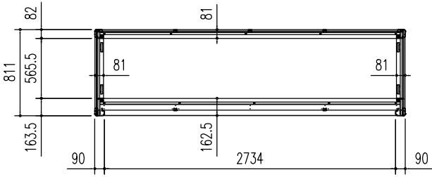
床 伏 図 (S = 1/50)
