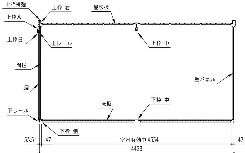
側面断面図 (S = 1/50)
