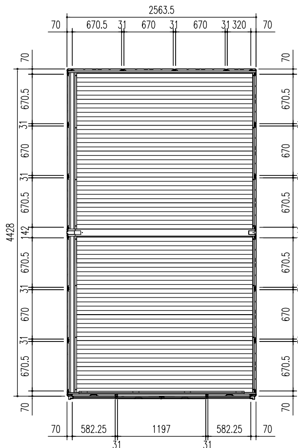
平面図 (S = 1/50)
