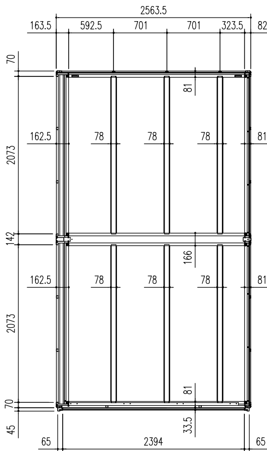
床伏図 (S = 1/50)
