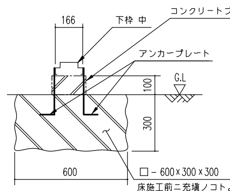
E ~ E' 断面 (内アンカー用)
