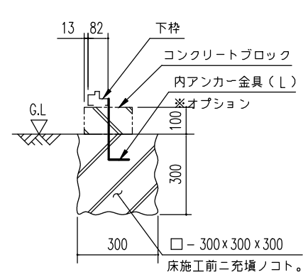
C ~ C' 断面 (内アンカー用)
