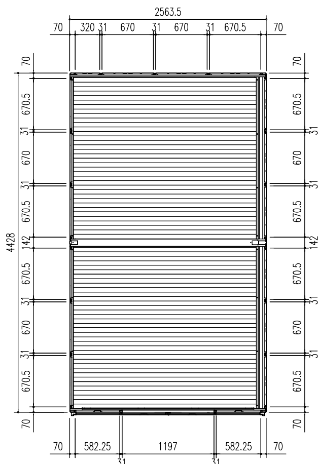
平面図 (S = 1/50)
