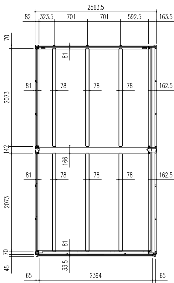
床伏図 (S = 1/50)
