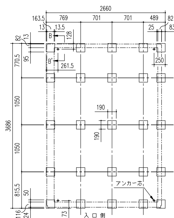
ブロック基礎伏図 (S = 1/50) (内アンカー用)
