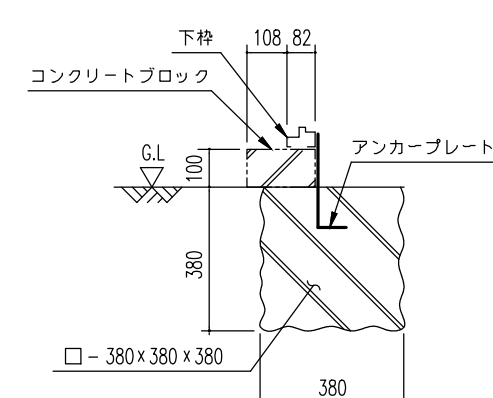
C ~ C'断面 (外アンカー用)
