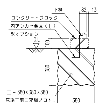
B ~ B'断面 (内アンカー用)
