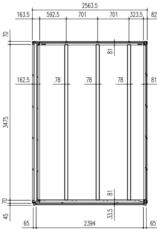
床伏図 (S = 1/50)
