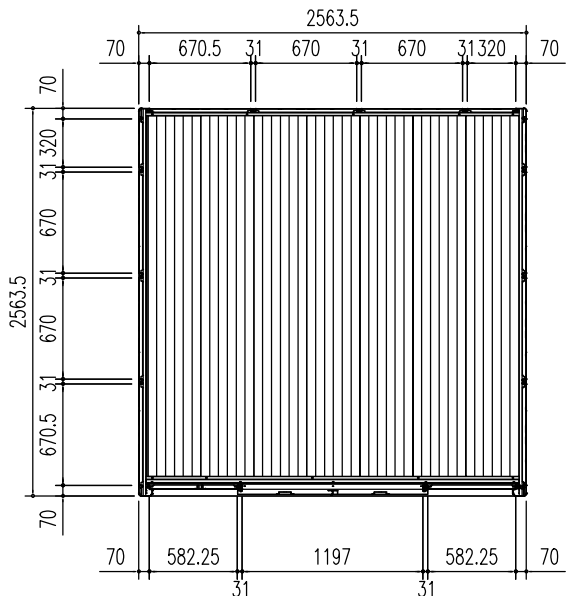
平面図 (S = 1/50)
