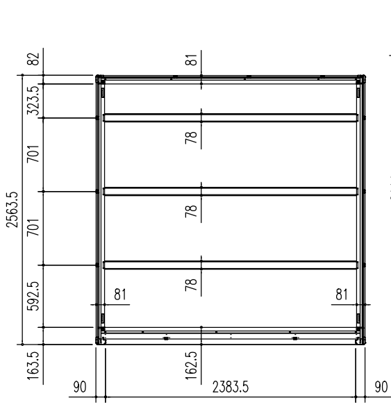
床伏図 (S = 1/50)
