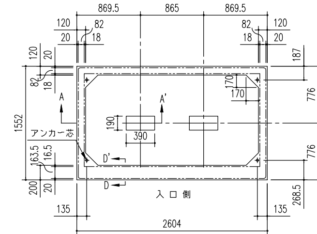
布基礎伏図 (S = 1/50)
