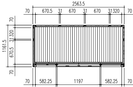
平面図 (S = 1/50)
