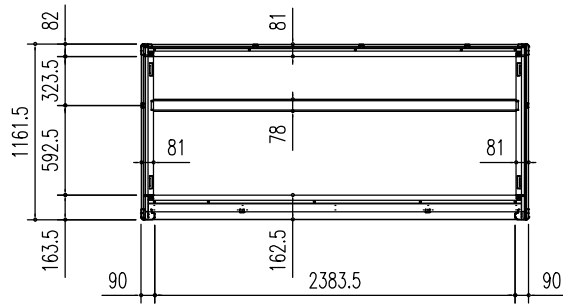
床 伏 図 (S = 1/50)
