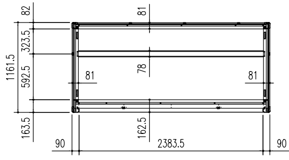
床 伏 図 (S=1/50)
