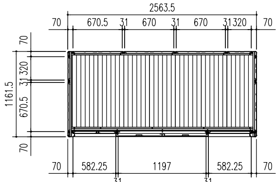
平面図 (S=1/50)
