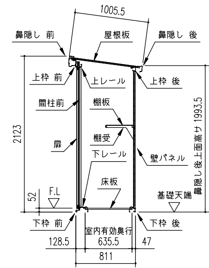
一般型矩計図 (S = 1/50)
