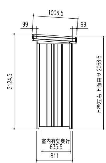
側面立面図 (S = 1/50)
