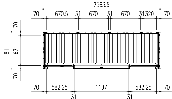
平面図 (S = 1/50)
