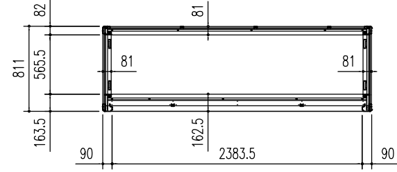
床伏図 (S = 1/50)
