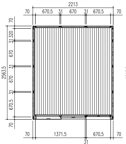
平面図 (S=1/50)
