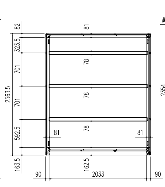
床伏図 (S=1/50)
