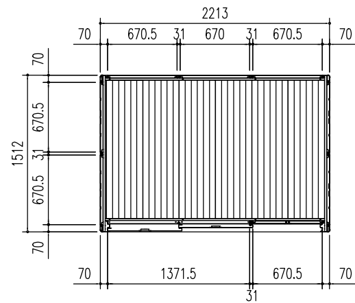
平面图 (S = 1/50)
