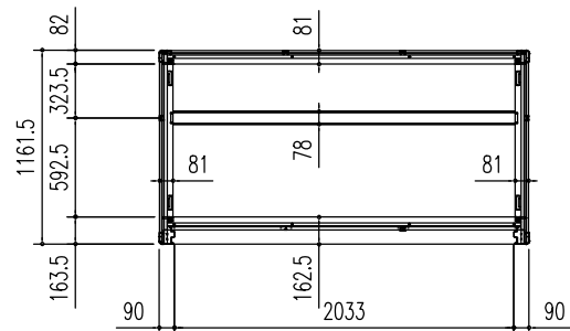
床伏図 (S=1/50)
