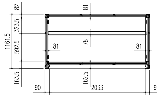
床伏図 (S=1/50)
