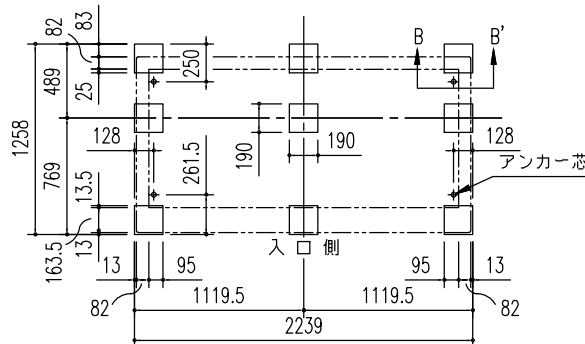
ブロック基礎伏図 (S=1/50) (内アンカー用) ※内アンカーセット(オプション) 別途必要
