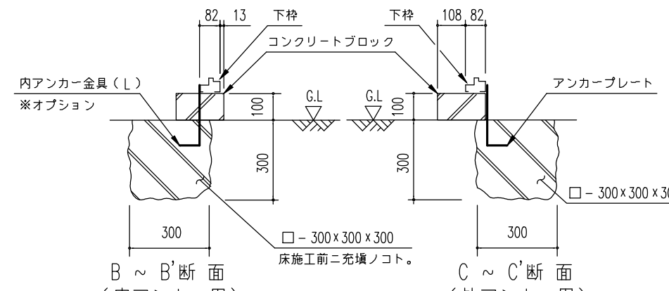
ブロック基礎断面図例 (S=1/20)
