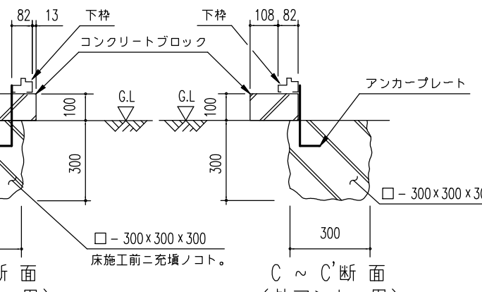
ブロック基礎断面図例 (S=1/20)
