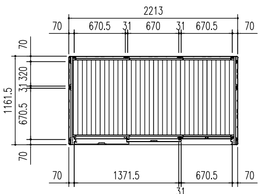
平面図 (S=1/50)
