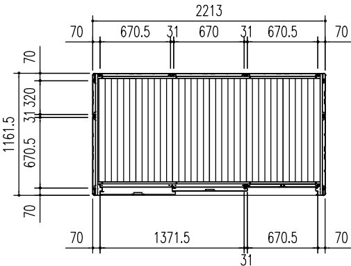
平面図 (S=1/50)
