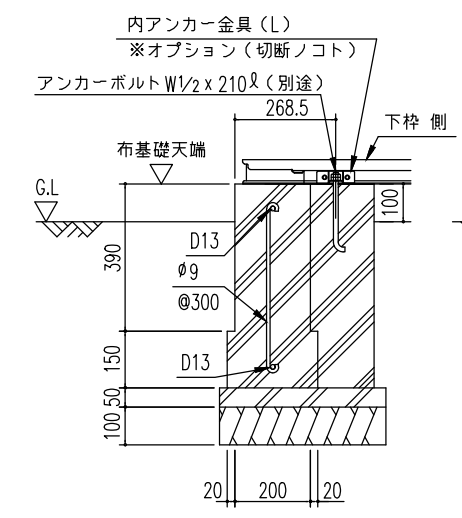
D ~ D'断面
