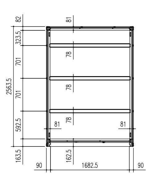
床伏図 (S=1/50)
