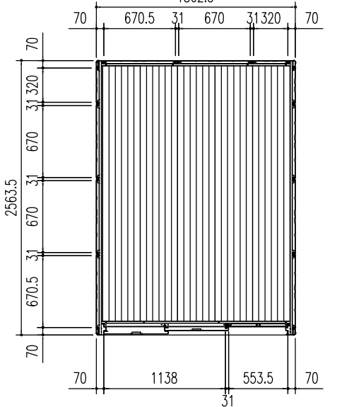
平面図 (S=1/50)
