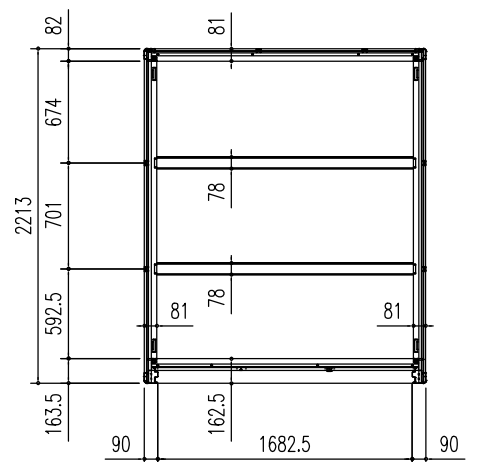
床伏図 (S=1/50)
