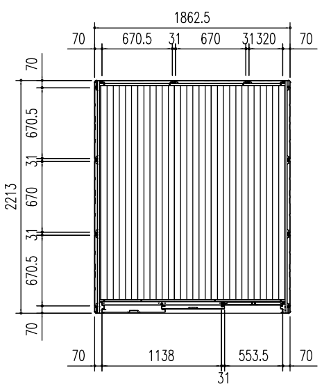
平面図 (S=1/50)
