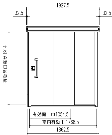
正面立面図 (S=1/50)
