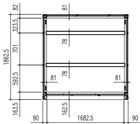
床伏図 (S=1/50)
