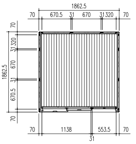
平面図 (S=1/50)
