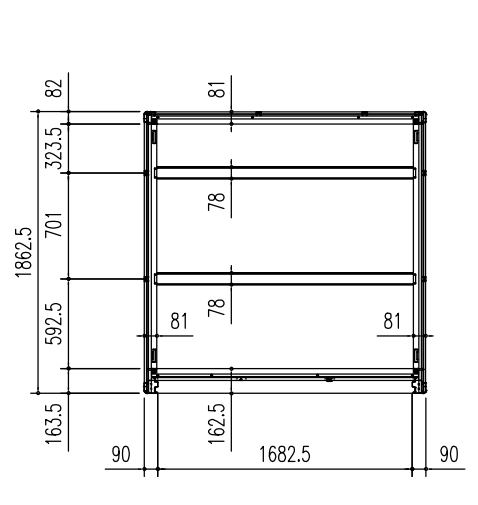
床伏図 (S=1/50)
