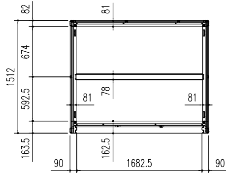
床伏図 (S=1/50)
