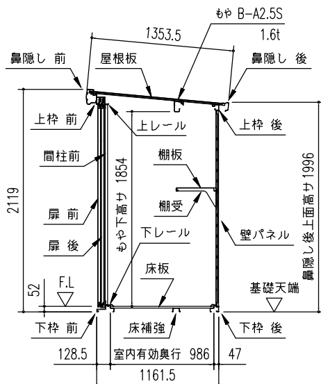
積雪型矩計図 (S=1/50)
