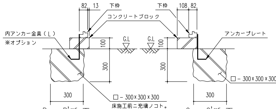
B ~ B'断面 (内アンカー用) C ~ C'断面 (外アンカー用) ブロック基礎断面図例 (S=1/20)
