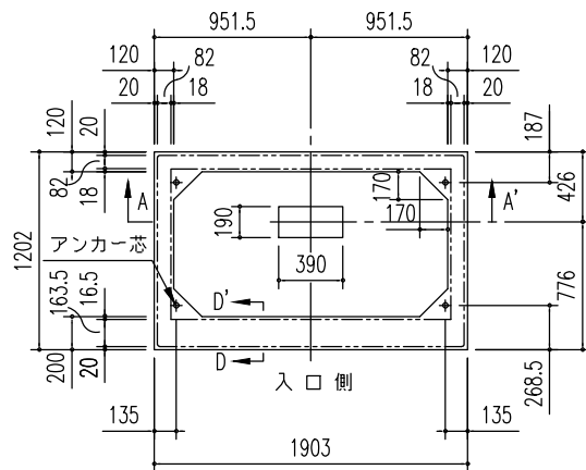
布基礎伏図 (S=1/50)
