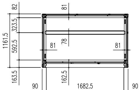
床伏図 (S=1/50)
