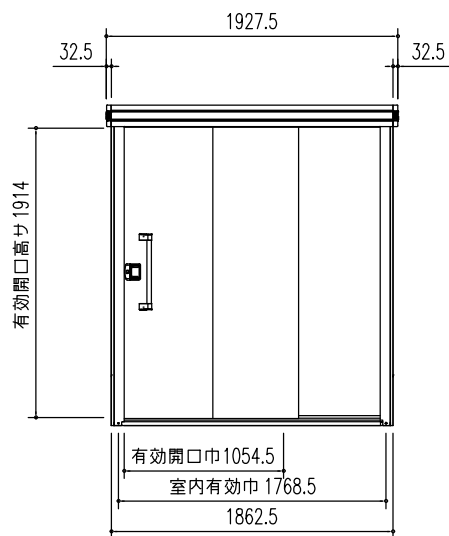
正面立面図 (S=1/50)
