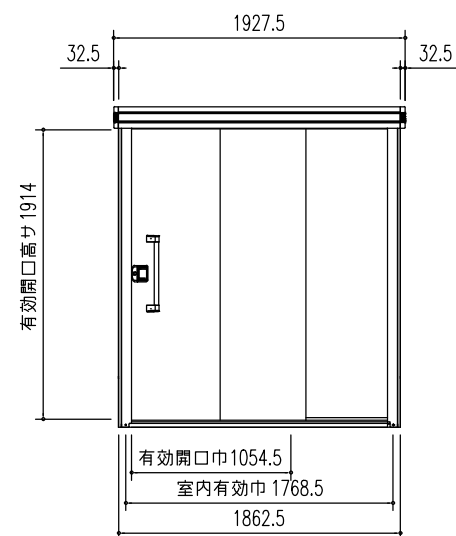
正 面 立 面 图 (S = 1/50)
