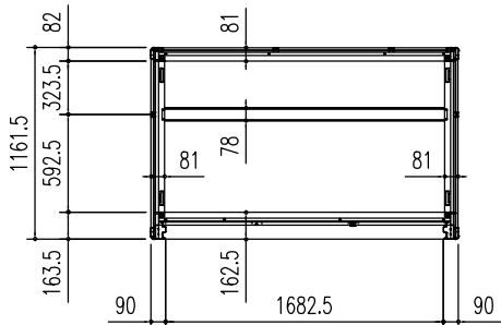
床伏図 (S=1/50)
