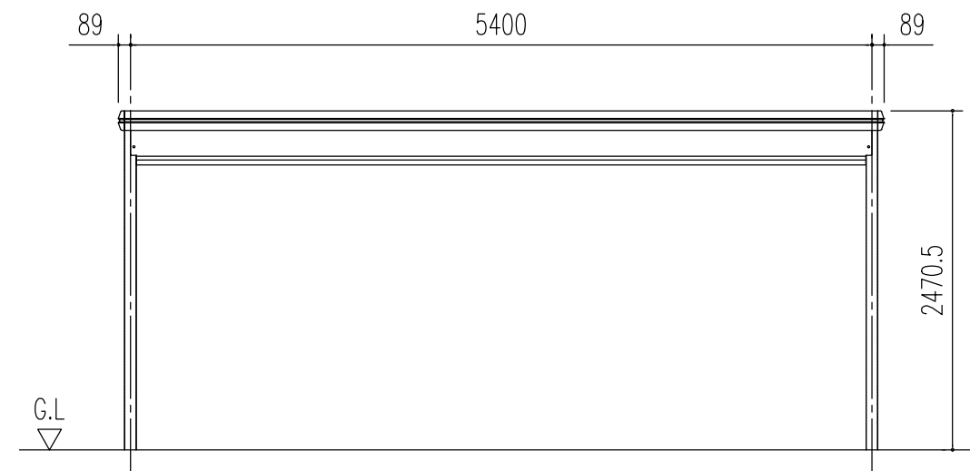
正面立面図 (S=1/50)
