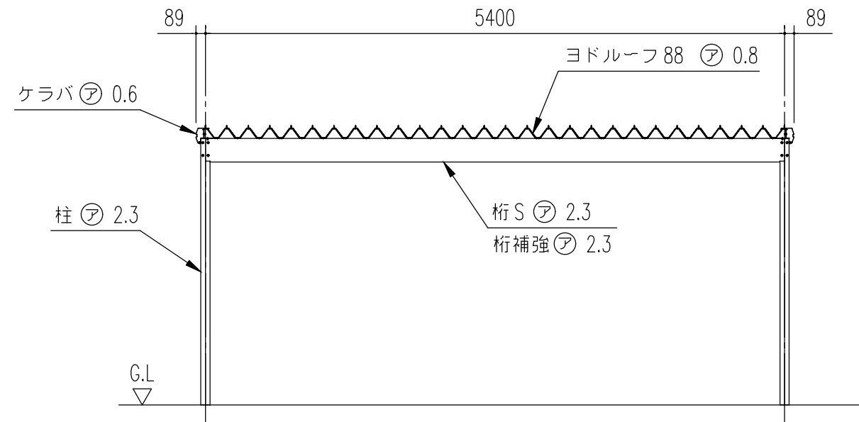
正面断面図 (S=1/50)
