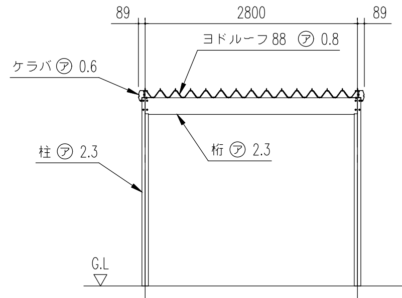
正面断面図 (S=1/50)
