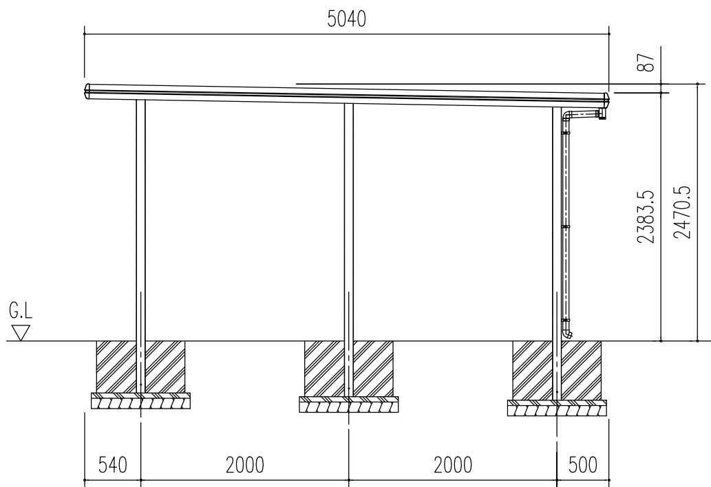
側面立面図 (S=1/50)
