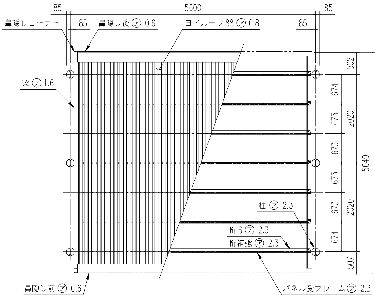
小屋伏図 (S=1/50)
