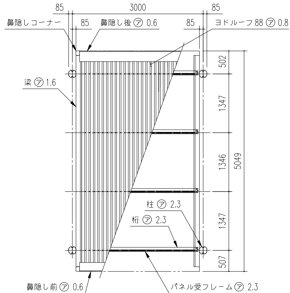
小屋伏図 (S=1/50)
