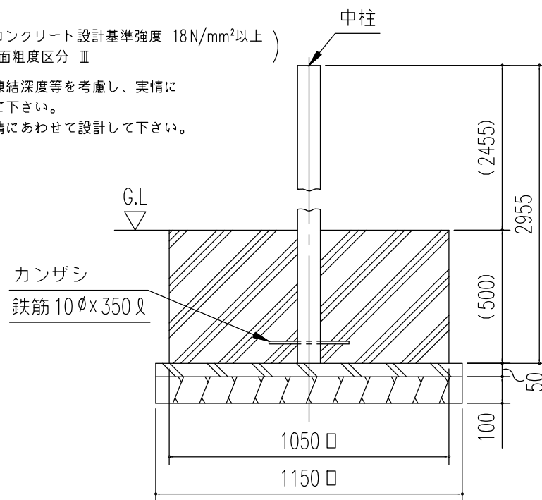
B ~ B' 断面 ベース筋 4-D13 x 4-D13
