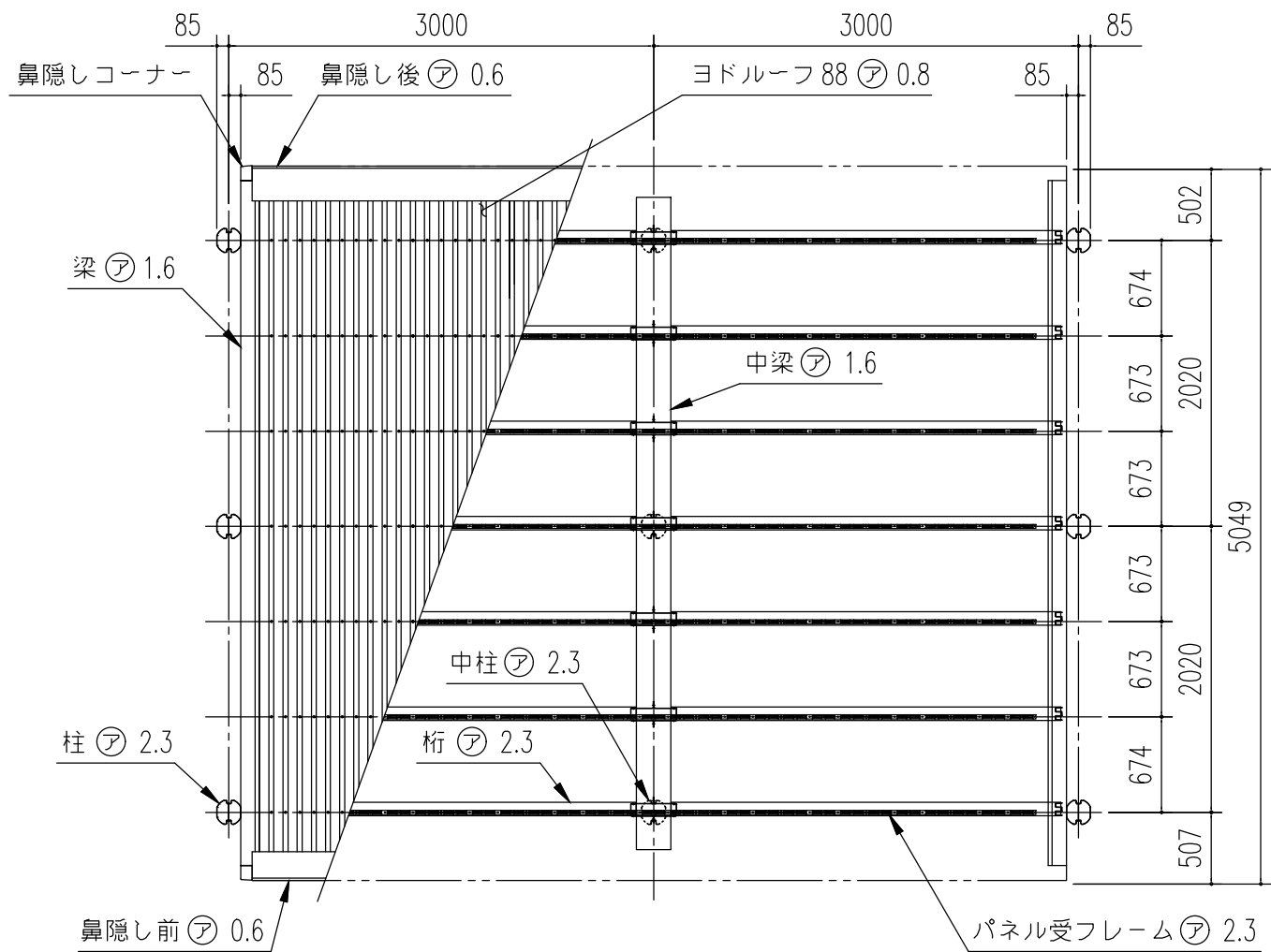
小屋伏図 (S=1/50)
