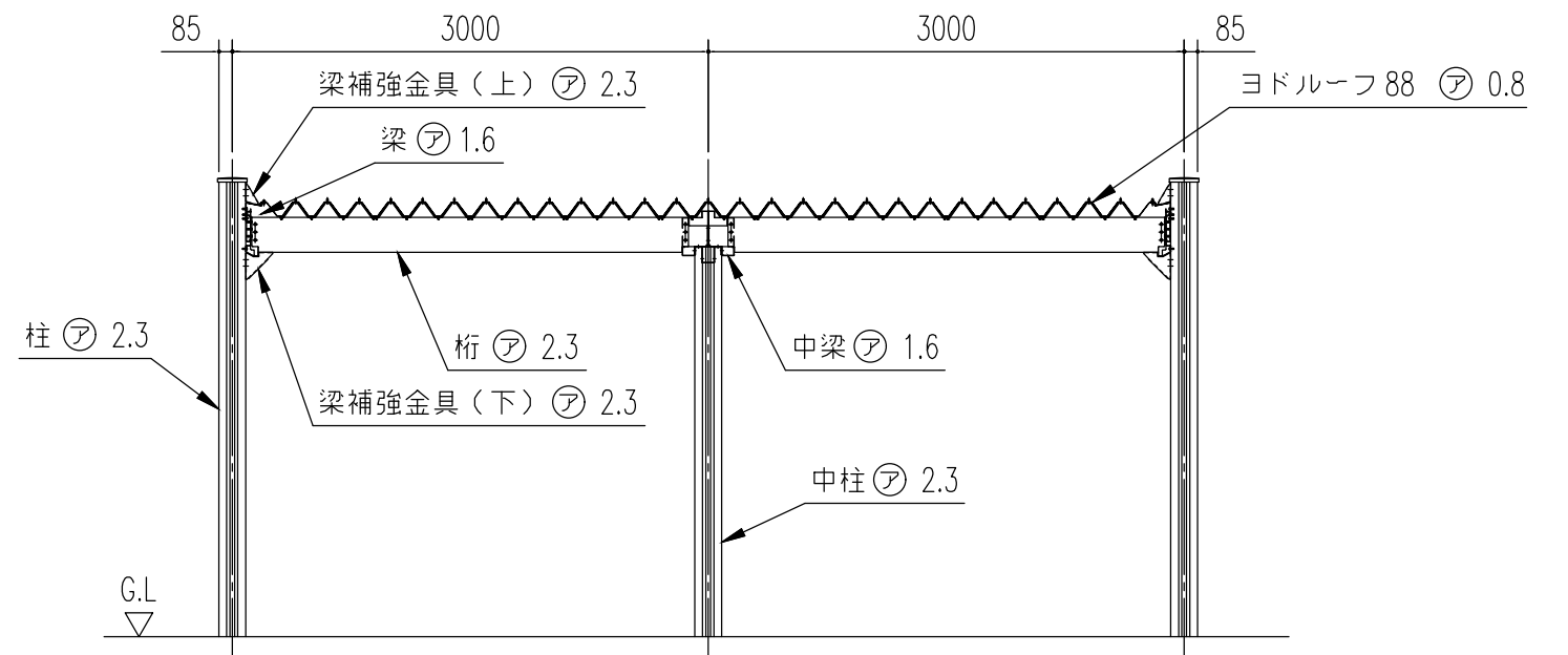
正面断面図 (S=1/50)
