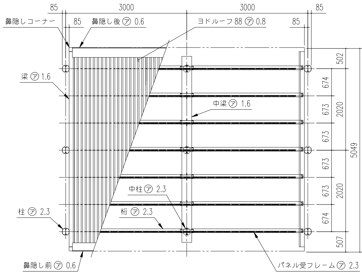
小屋伏図 (S=1/50)
