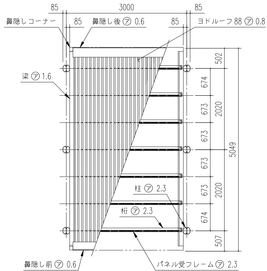
小屋伏図 (S=1/50)
