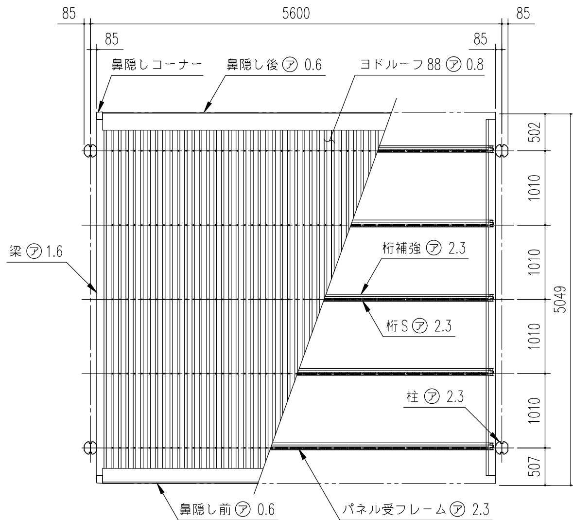
小屋伏図 (S=1/50)
