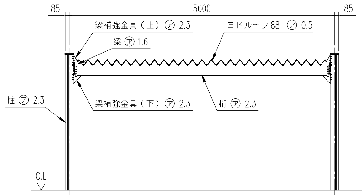
正面断面図 (S=1/50)
