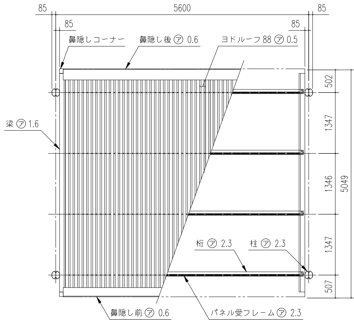
小屋伏図 (S=1/50)
