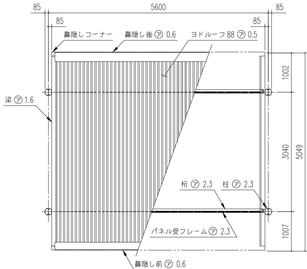
小屋伏図 (S=1/50)
