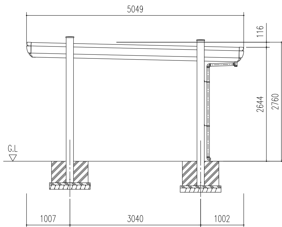
側面立面図 (S=1/50)
