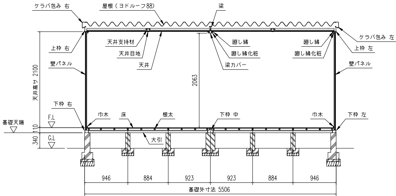
正面断面図 (S=1/50)
