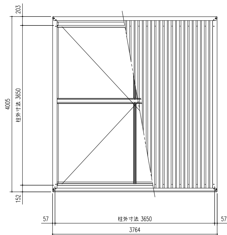
前 小屋伏せ図 (S=1/50)
